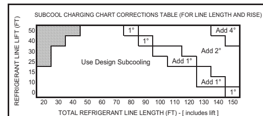
060J, 060K & 061C Units
