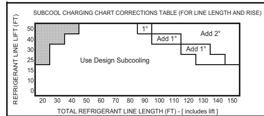
035J, 036J & 041J Units
